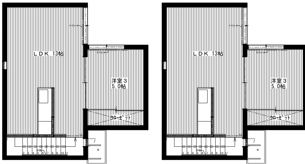
【2階平面図】
